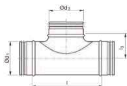
OBJT (TCPU) - lisovaná
