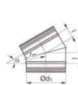
oblouk OST (BFU) 30°
