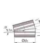
oblouk OST (BFU) 15°
