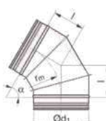
oblouk OST (BFU) 60°
