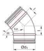
oblouk OLT (BU) 45°
