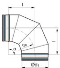
OST (BFU) - oblouk 90° (r=d) segmentová verze
