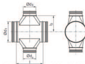
XCU - Odbočka oboustranná, s integrovaným sedlovým dílem, centrický, pozinkovaný
