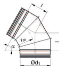
OST (BFU) - oblouk 60° (r=d) segmentová verze
