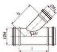
TVU - dbočka 45°, pozink, segment
