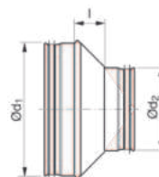
PROLT (RCU) - lisovaná verze
