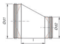
PRET (RLU) - pozink, excentrická, segmentová
