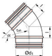
OLT (BU) - oblouk 45° (r=d) lisovaná verze
