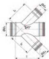
XVU - dvojtá odbočka 45°, pozink
