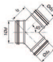
YVU - rozdělení v úhlu 45°
