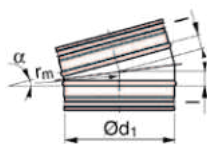
OST (BFU) - oblouk 15° (r=d) segmentová verze
