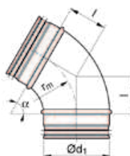
OLT (BU) - oblouk 60° (r=d) lisovaná verze
