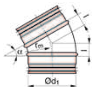
BOLT (BU) - oblouk 30° (r=d) lisovaná verze
