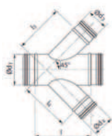
XVU - dvojitá odbočka 45°, pozink
