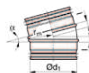
OLT (BU) - oblouk 15° (r=d) lisovaná verze
