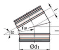
OST (BFU) - oblouk 30° (r=d) segmentová verze
