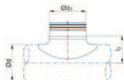
SDLT (PSU) - lisované provedení (s optimalizovaným poloměrem proudění)
