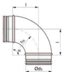
OLT (BU) - oblouk 90° (r=d) lisovaná verze
